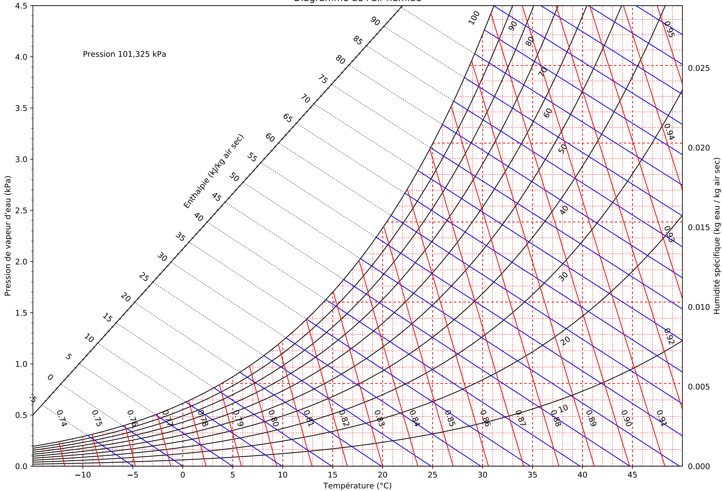
Diagramme de l'air humide
